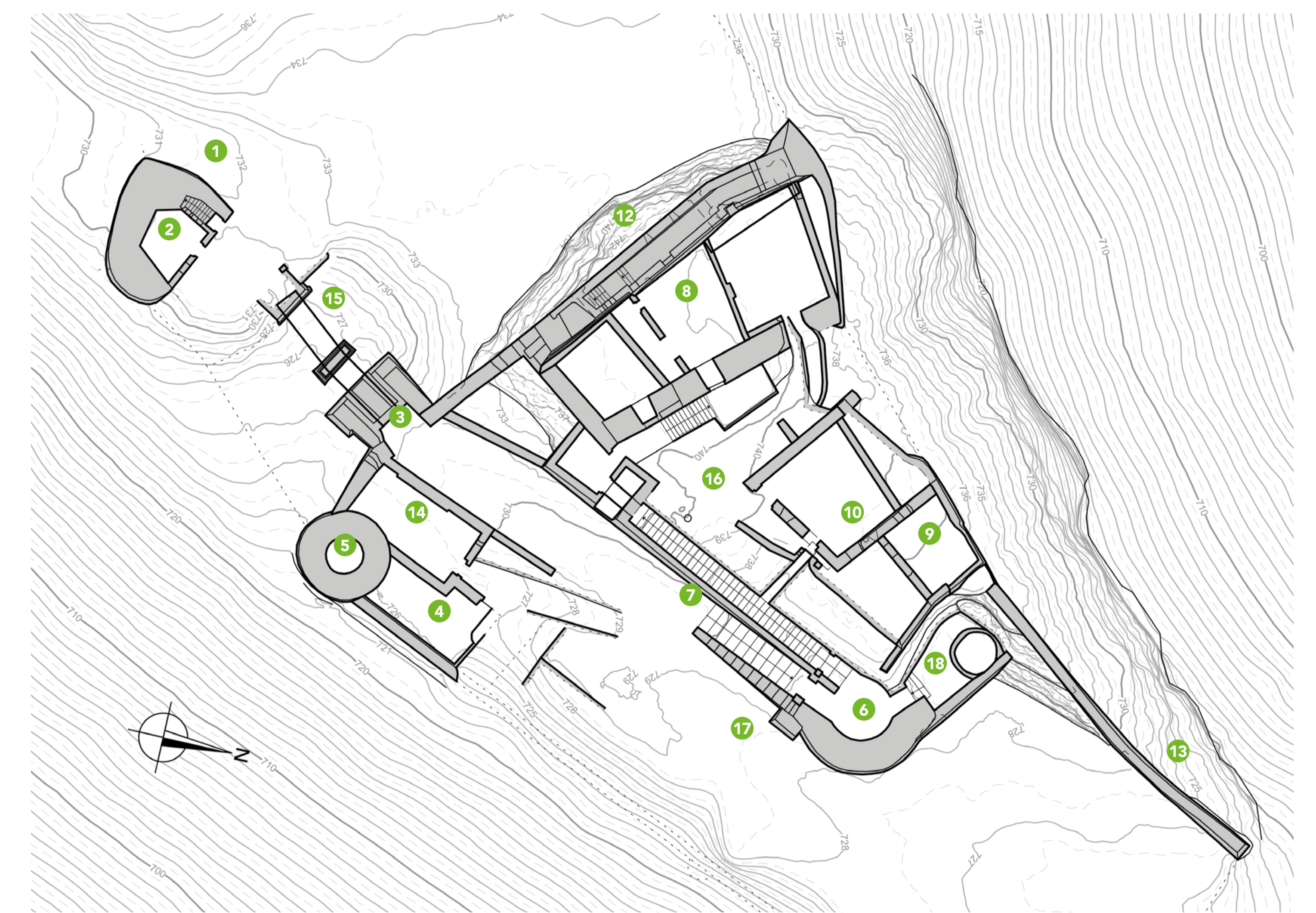
Die Farnsburg im Mauergrundriss und mit Höhenkurven; deutlich zeigt sich, dass der Ostteil der Unterburg noch grösstenteils intakt ist. Für die Bezeichnung siehe Legende auf der Rekonstruktion links (Plan: Terradata AG, Einsiedeln).
