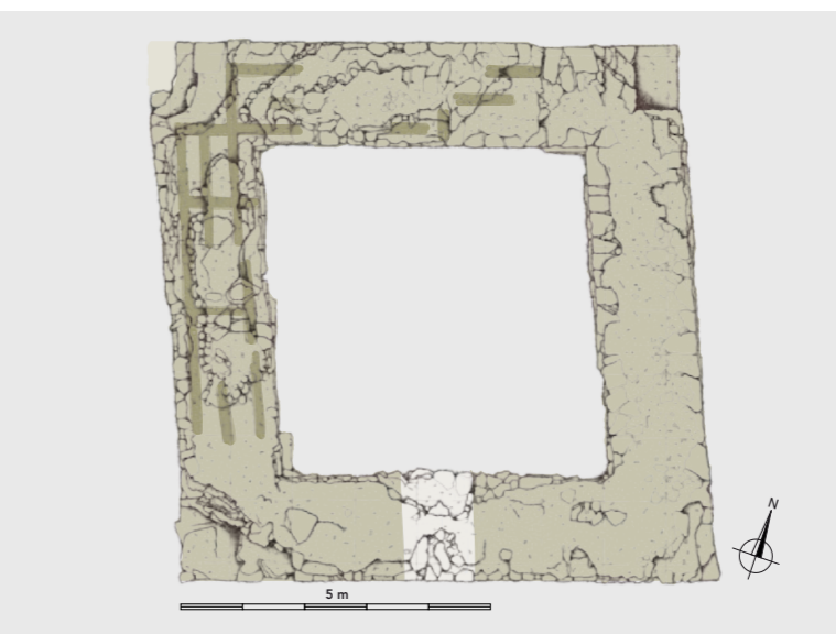
Der Grundriss des Wachturms in Muttenz: Die durch die vergangenen Holzbalken entstandenen Hohlräume sind dunkler eingefärbt, die mutmassliche Türöffnung ist hell dargestellt.
